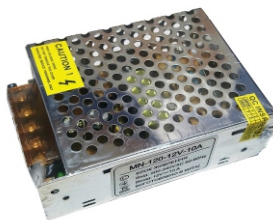
55532 Блок живлення MN-120-12 120W 10A AC180-264 негерметичний Compact IP20
