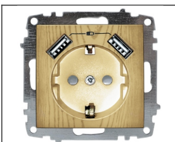
13582 Розетка ZENA 1-а з заземленням + шторки +2-а USB розетка береза/клен (модуль)
