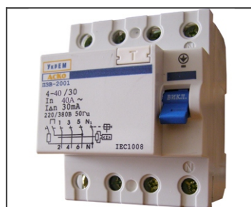
07136 Пристрій захисного відключення ПЗВ-АСКО-2001 4р/ 40А/ 30mA
