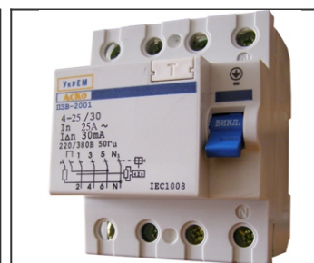
07132 Пристрій захисного відключення ПЗВ-АСКО-2001 4р/ 25А/ 30mA
